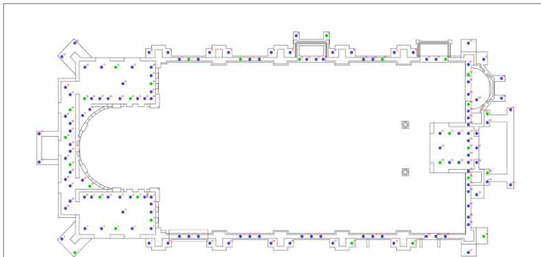
Dit is het palenplan van de restauratie van de St. Barnabaskerk.
